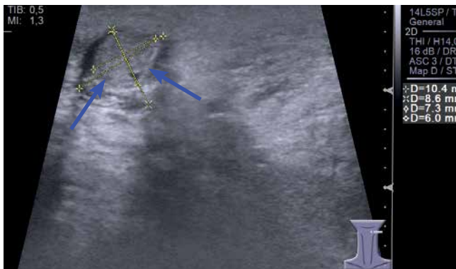
Рис. 5. Ультразвуковая томограмма. Опухоль левой небной миндалины (синие стрелки)
