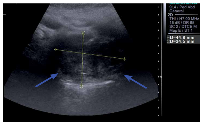
Рис. 2. Ультразвуковая томограмма. Внеоргannая опухоль парафарингеального пространства (синие стрелки)
