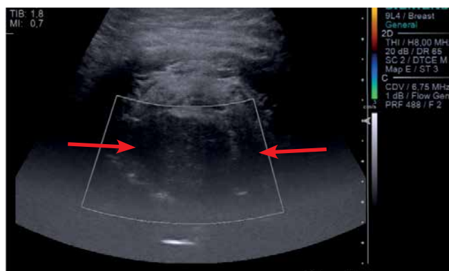
Рис. 1. Ультразвуковая томограмма. Эктопированная щитовидная железа в область корня языка (красные стрелки)
