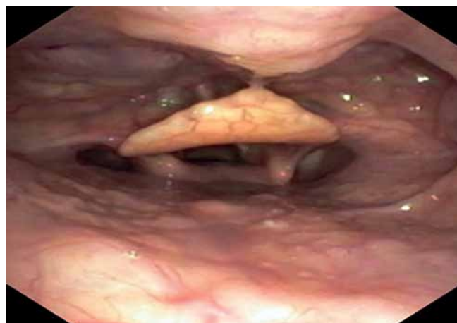
Рис. 7. Эндоскопическое исследование ротоглотки. Слизистая в области корня языка не изменена
