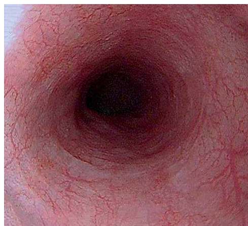
Рис. 5. Визуальный контроль спустя 1 мес Fig. 5. Visual control 1 month after stenting
